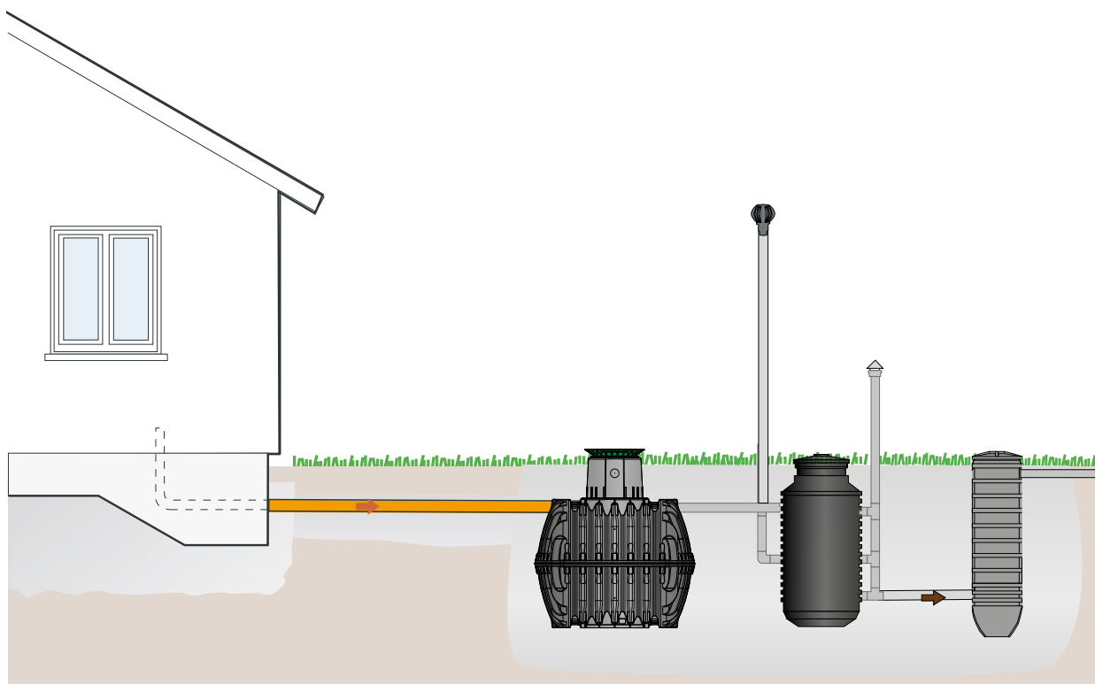
Installationsförslag, Conclean kompakt markbädd med pumpstation
